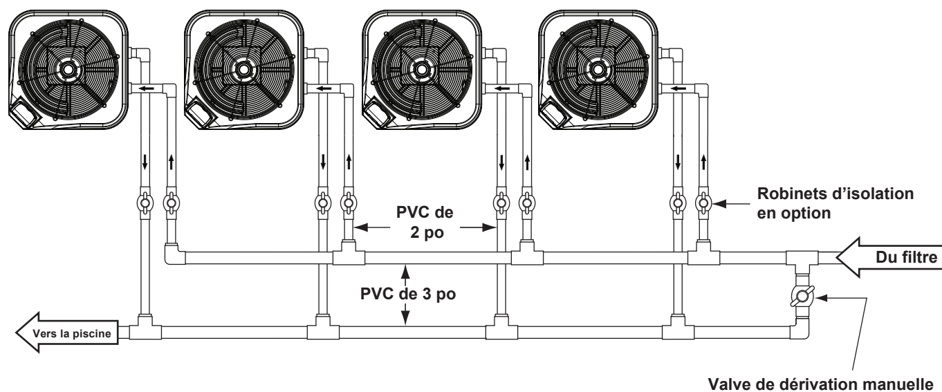
Figure 7. Disposition de la plomberie de quatre (4) thermopompes
