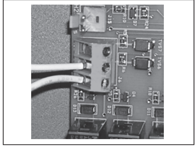
Figure 10b. Connexion AquaLink RS ou connexion à distance TSTAT (Connexion à 2 fils)
