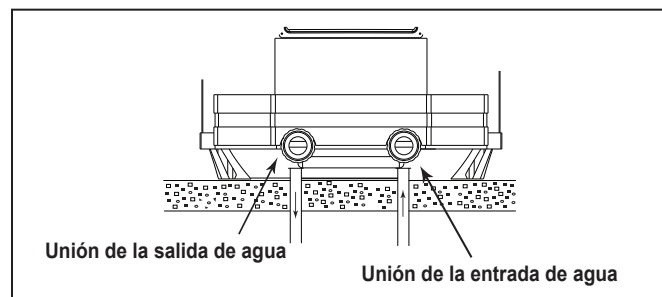
Figura 15. Preparación de la bomba de calor JE para el invierno
