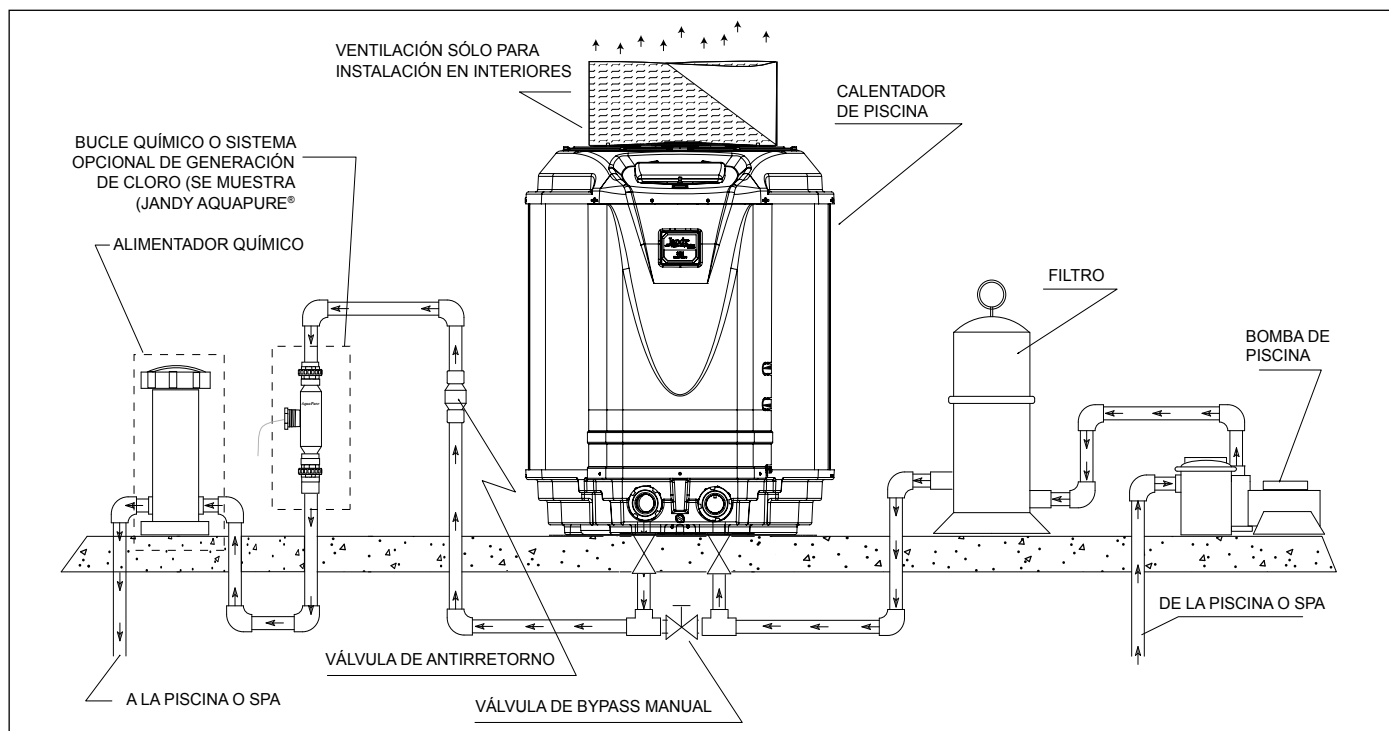
Figura 4. Distribución hidráulica estándar
