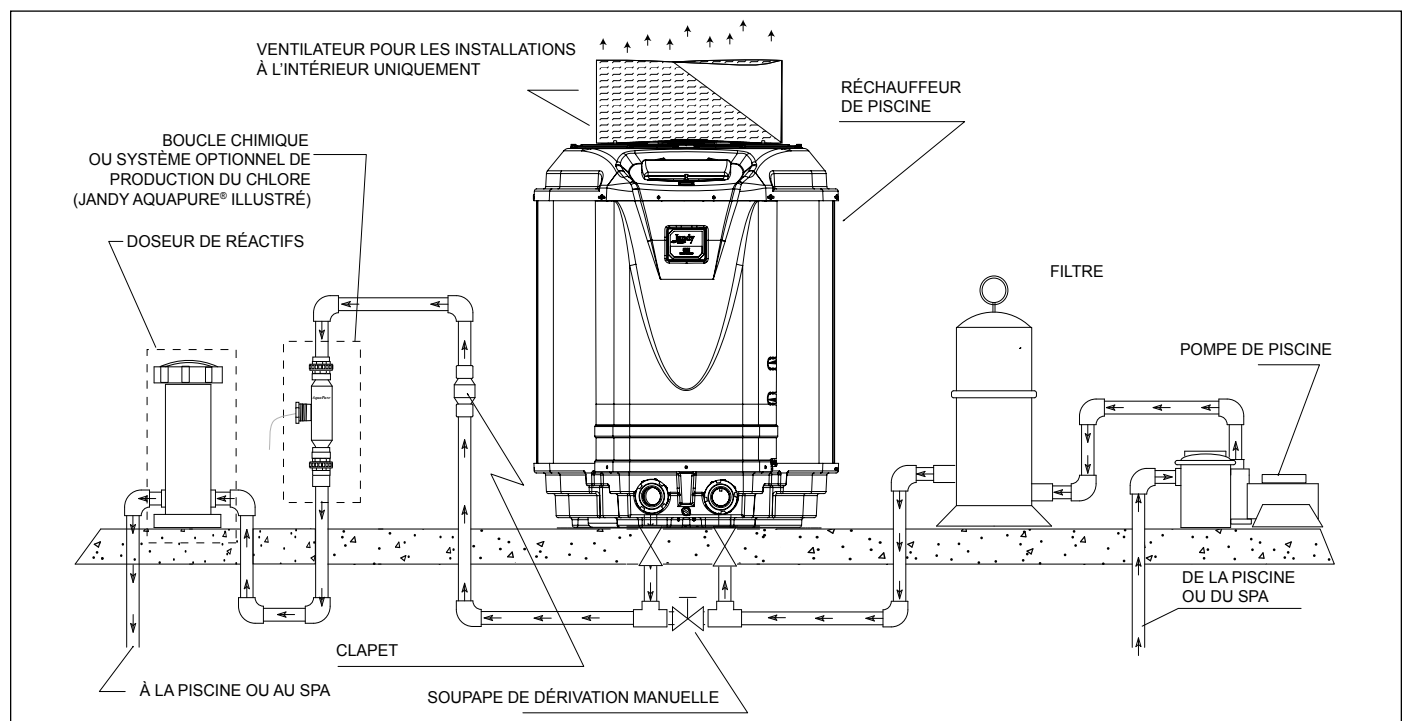
Figure 4. Disposition de la plomberie standard
