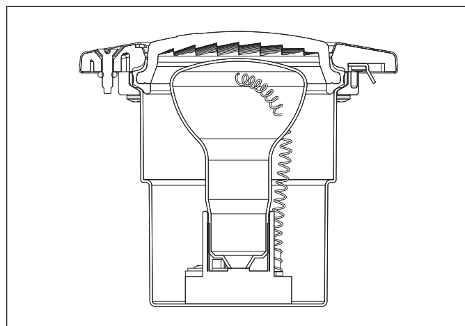
Figure 14. Vue en coupe de la lampe blanche de spa Jandy
