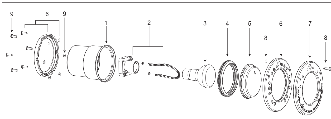
Figure 12. Lampe blanche de spa Jandy, vue éclatée
