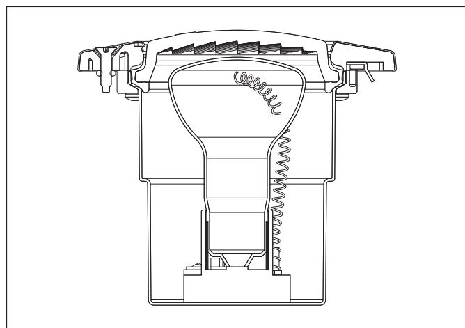
Figura 14. Plano transversal de la luz blanca Jandy para spas
