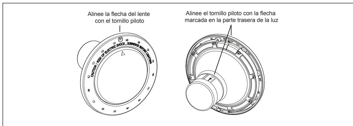
Figura 8. Alineación del lente, el aro frontal, el compartimento y las abrazaderas de las luces blancas para piscinas
